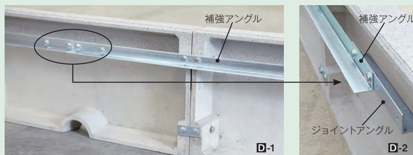
2本の「補強アングル」同士を、「ジョイントアングル」で連結します。
