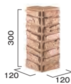
コバ 135° 出隅
