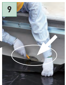
9 水がパネル外に抜けるように、耐根補助シートに切り込みを入れます。
