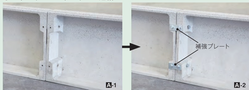
連結部ボルト締め (仮締め)
