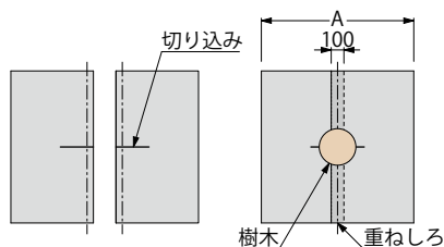
寸法表〔丸型〕 &lt;単位:mm&gt;
